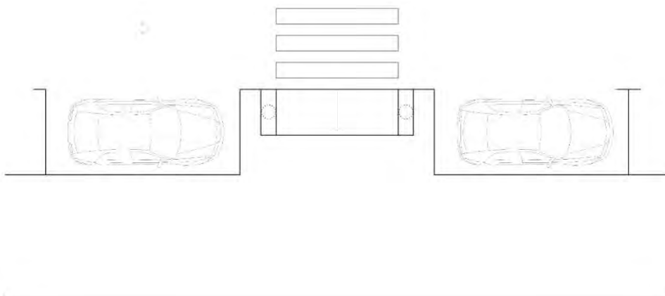
Ejemplo 12. Recomendaciones para la mejora de la visibilidad en el cruce. Avance del vado peatonal a la línea de aparcamiento y calzada.
