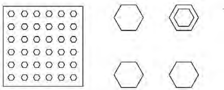
Ejemplo 32. Pavimento táctil indicador de advertencia con botones de forma funcionalmente equivalente a la troncocónica.
