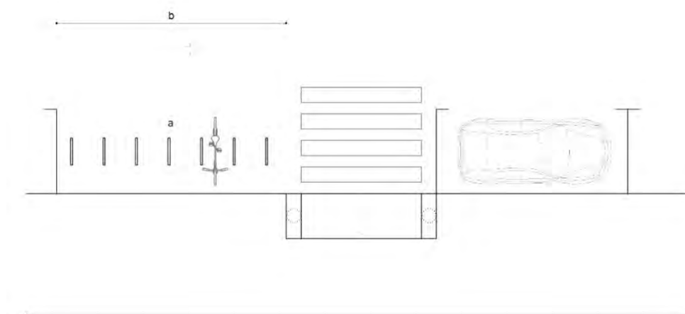
Ejemplo 11. Recomendaciones para la mejora de la visibilidad en el cruce, cuando el vado peatonal se mantiene en la línea de la acera.
