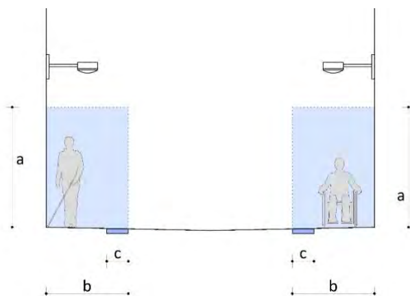
Ejemplo 5. Zona de plataforma única: delimitación del espacio de uso exclusivo peatonal mediante pavimento táctil
