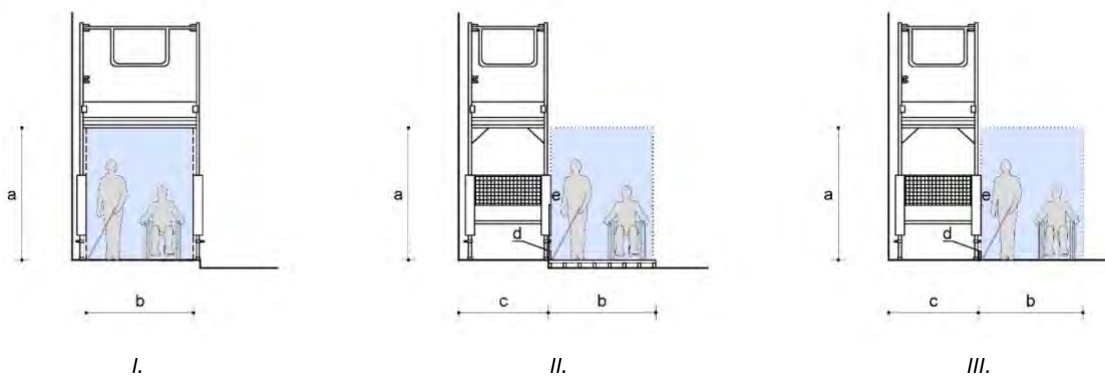
Ejemplo 28. Ejemplos para la configuración de IPAs en las obras e intervenciones (I. IPA por debajo del andamio; II. IPA sobre plataforma en la calzada; III. IPA paralelo al andamio).
