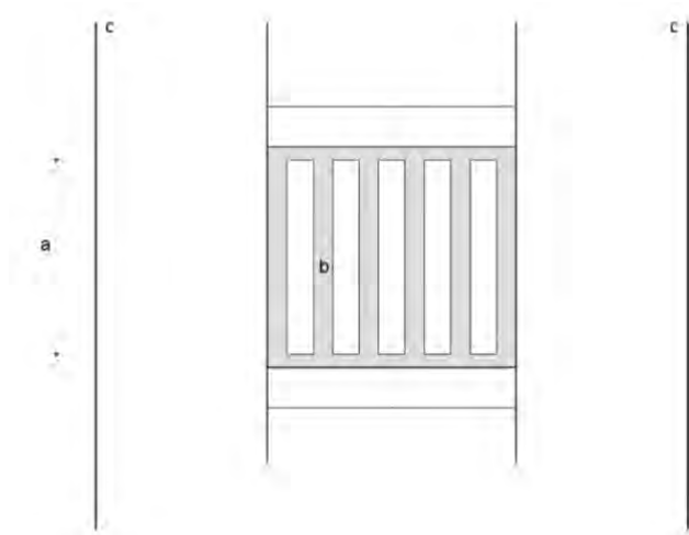
Ejemplo 16. Esquema gráfico de paso de peatones mediante elevación de la calzada al nivel de la acera.
