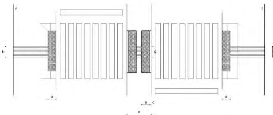
Ejemplo 38. Aplicación del pavimento táctil indicador en isleta nivelada con la calzada.
