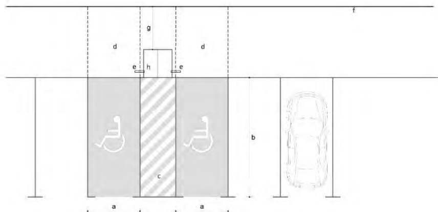
Ejemplo 25. Plaza de aparcamiento reservada dispuesta en perpendicular a la acera, con espacio de transferencia compartido.
